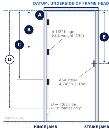
FRAME ELEVATION
